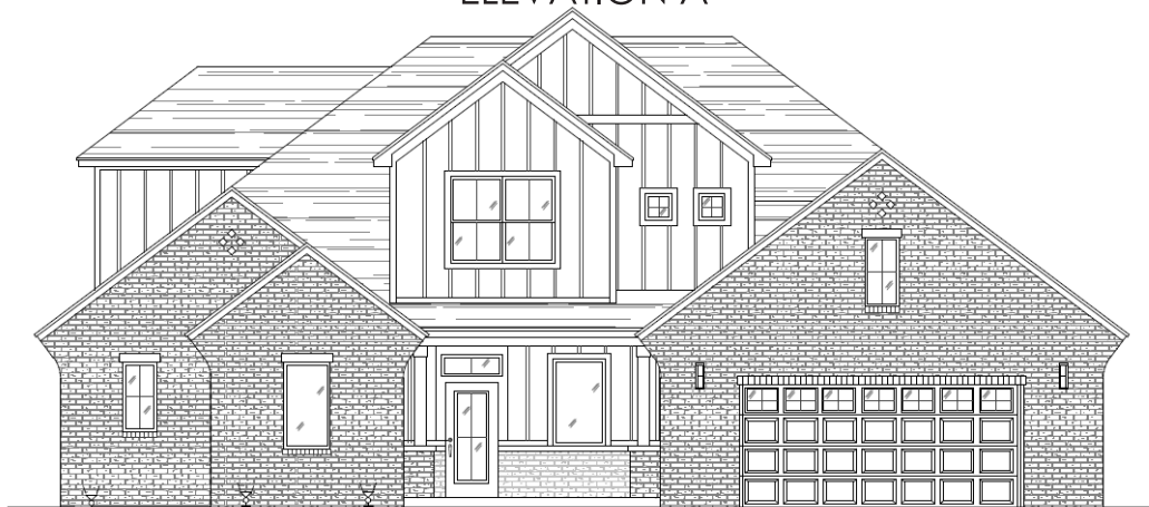
ELEVATION A
