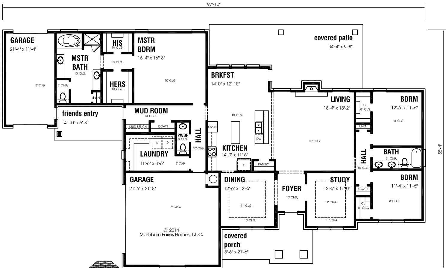
Elevation A
